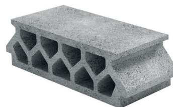
CZAMANINEK K9/16 60EU
