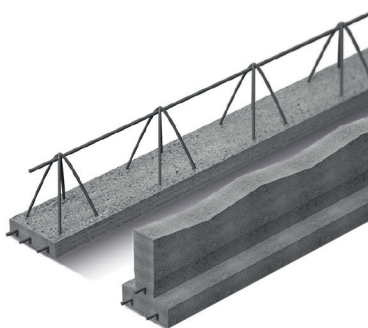
Belki klasyczne i sprężone
